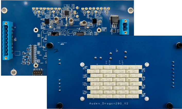
mmW Array Antenna Module
