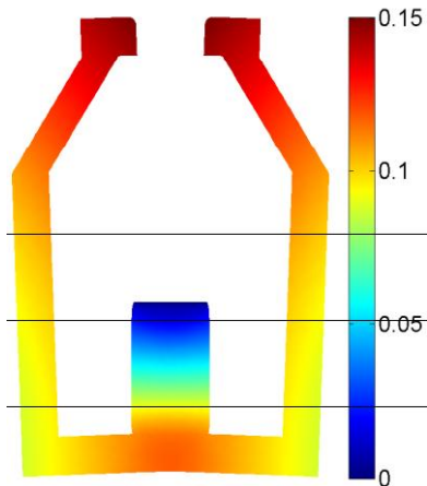
Piezoelectric Microgripper
